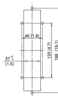
Схема отверстий малого корпуса
